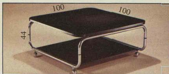
FLAMINGO ●möbelfakta 100x100 cm, höjd 44 cm. Skivor: Askfaner med polyuretanlack på tinterbrun lasyr. Underrede: Förkromade stälror, fyra klothjul. Monterbart. 30 kg. Miljö på sidan 54. Krom/tinterbrun ask kr ..... 378:–
